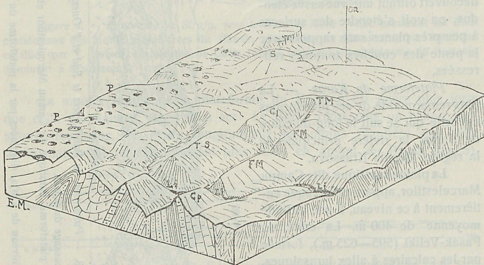
Figure 2. — Block diagramme des crêtes à inversion de relief
