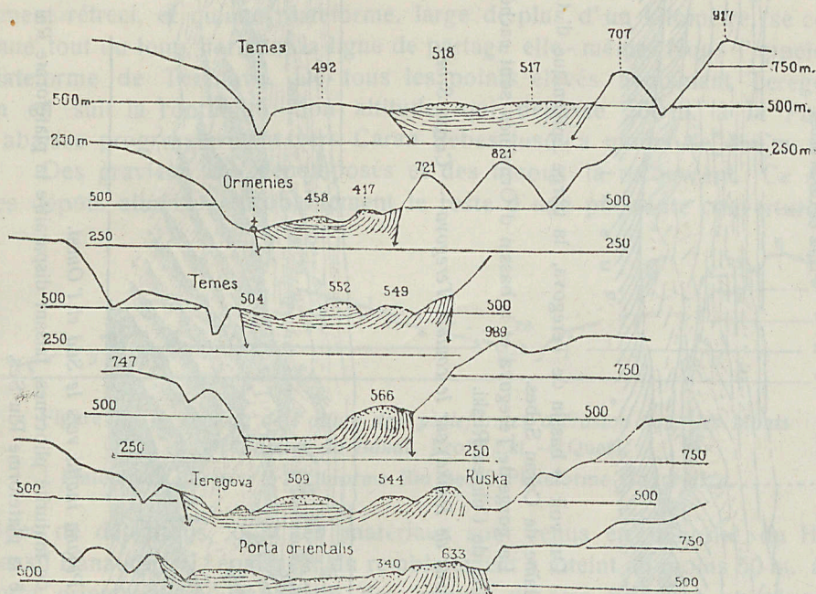
Figure 7. — Série de profils Est — Ouest du couloir Caran Sebes — Porta Orientalis, montrant le fossé tectonique et les gorges épigéniques.
