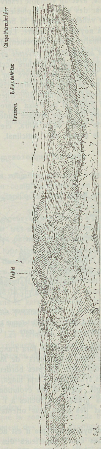
Figure 3. — Panorama du Pasak, vers le Sud et l' Ouest.
