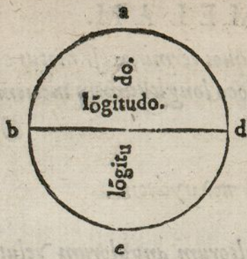
Triangulus æquilaterus
