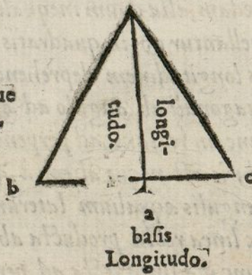
Triangulus trium inæqualium laterum.
